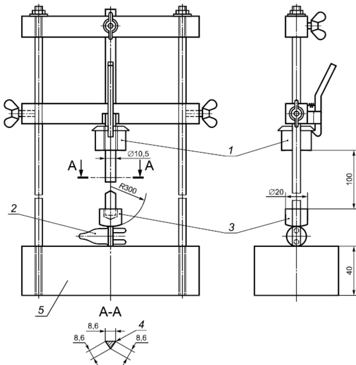
1 - боек массой (1000±2) г; 2 - образец; 3 - прижим массой 100 г; 4 - края закруглить; 5 - стальная опора (10±1) кг Рисунок 27 - Устройство для проверки механической прочности розеток, вилок, разветвителей и удлинителей
