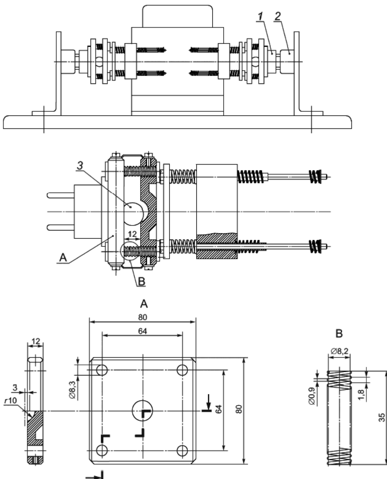
1 - вилка; 2 - розетка; 3 - стальной шар
