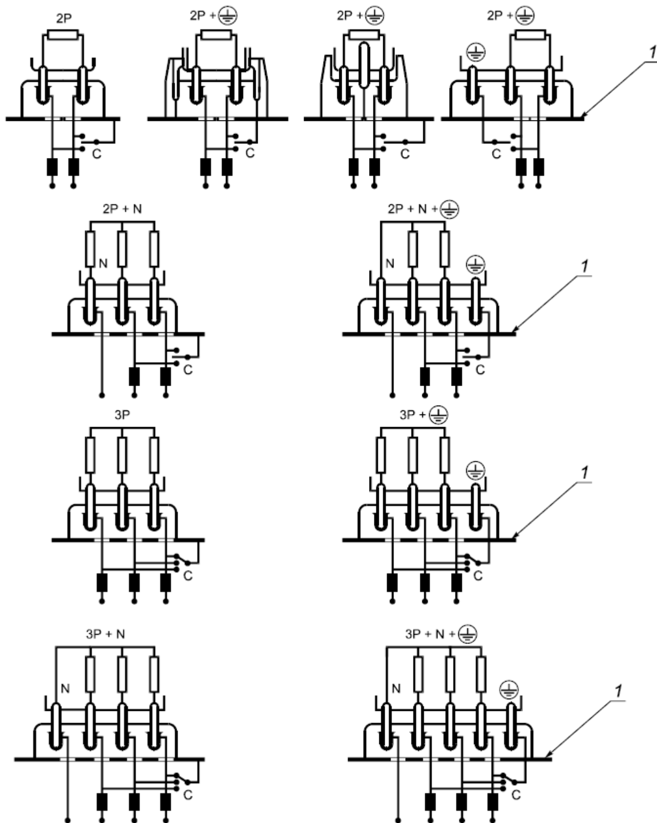
Рисунок 17 - Схема соединения для испытания на нормальную работу
