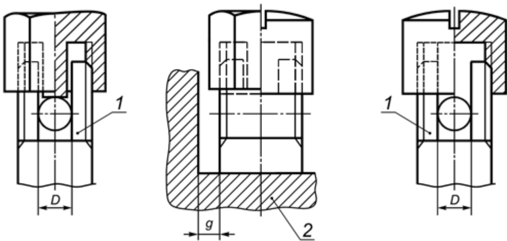
Рисунок 4 - Зажим с прижимной планкой
