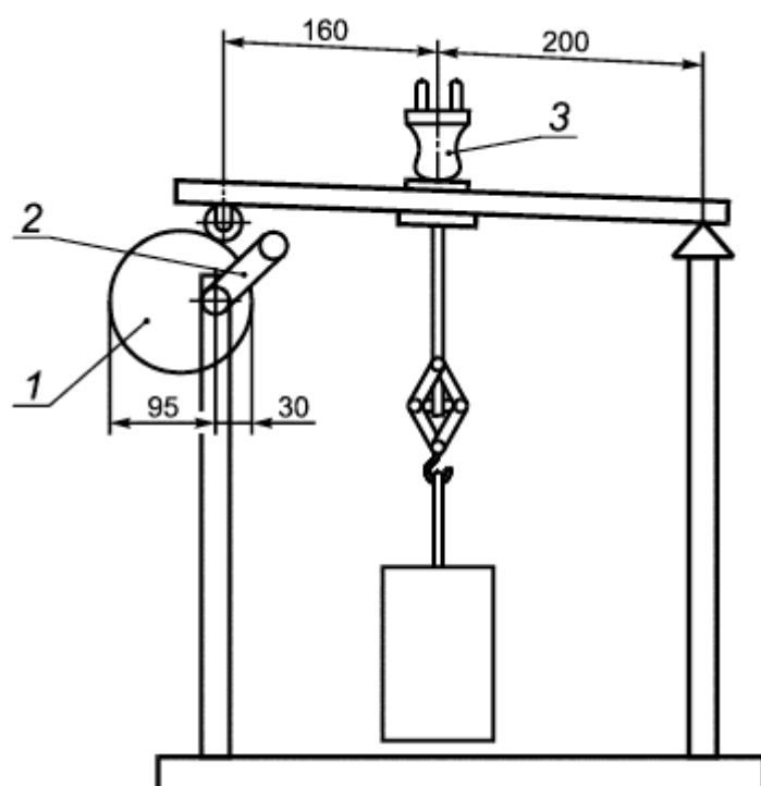
Рисунок 20 - Установка для испытания узла крепления шнура
