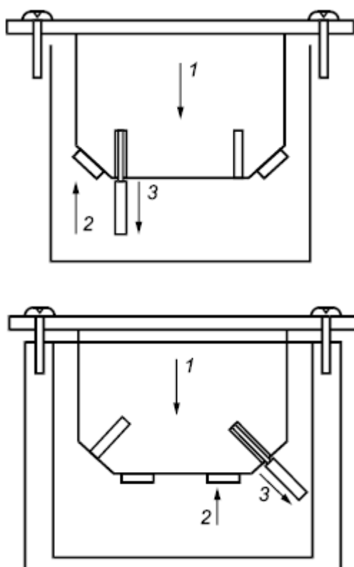
а) определение направления приложенных сил 1 - направление монтажа; 2 - направление силы, приложенной на подсоединение и отсоединение (120 Н); 3 - направление для вытягивания проводника 30 Н в течение 1 мин Рисунок 46, лист 1 - Проверка требований 13.4
