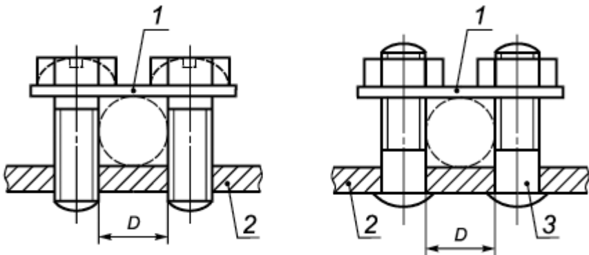
Рисунок 3 - Зажимы с крепежной головкой и гайкой
