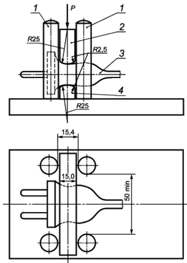
1 - направляющие; 2 - подвижный зажим; 3 - образец; 4 - неподвижный зажим; P - направление приложения силы Рисунок 38 - Установка для испытания на сжатие вилок
