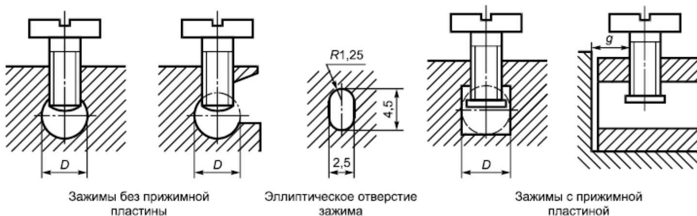
Рисунок 1 - Пример соединителей
