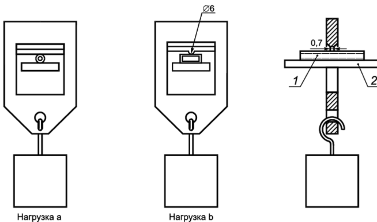
Рисунок 41 - Установка для испытания давлением при высокой температуре
