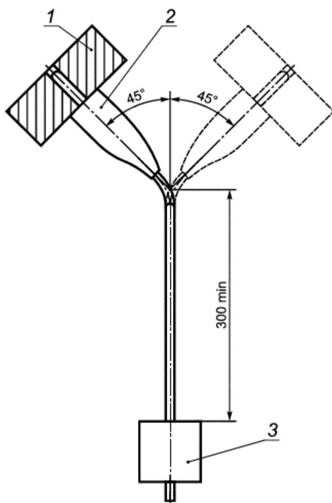
Рисунок 20 - Установка для испытания узла крепления шнура
