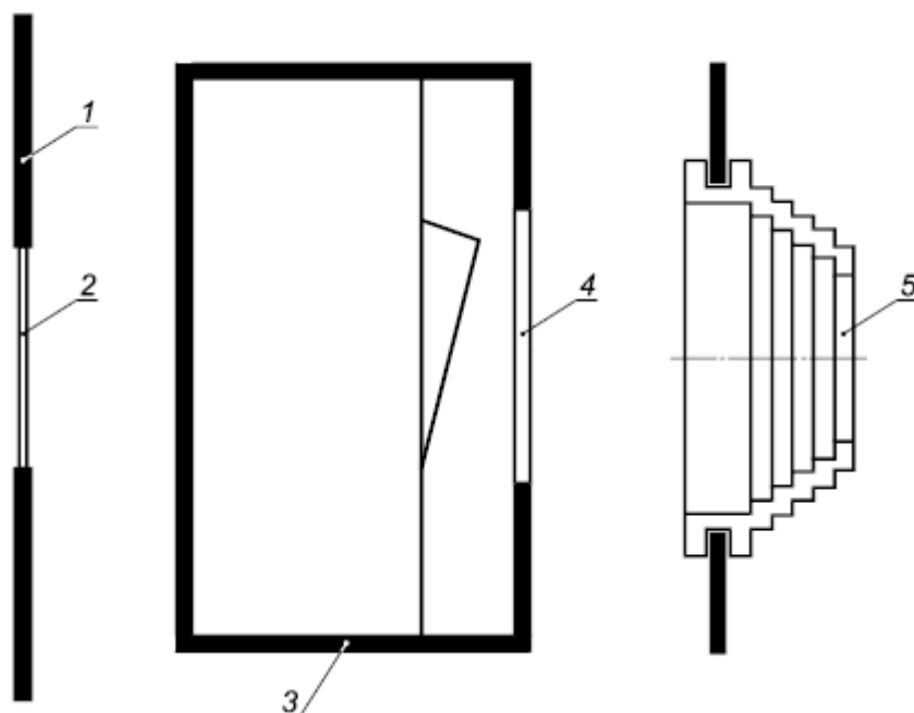
1 - оболочка; 2 - входная мембрана; 3 - конверт; 4 - защитная мембрана; 5 - кабельный ввод Рисунок 45 - Примеры мембран и прокладок
