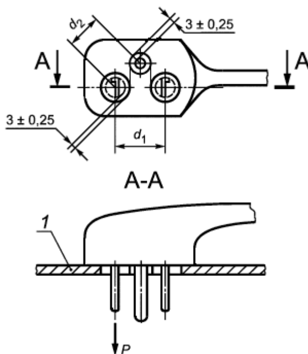
Рисунок 30 - Устройство для проверки механической прочности вилок
