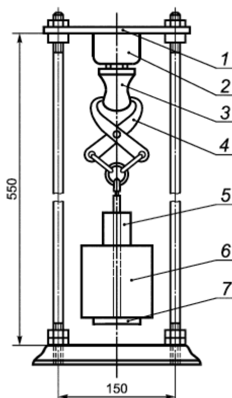
1 - держатель; 2 - образец; 3 - испытываемая вилка; 5 - захват; 6 - основной груз; 7 - опора Рисунок 18 - Установка для проверки усилия разъема штырей вилки с гнездами розетки
