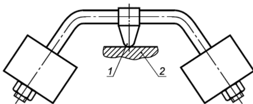
Рисунок 37 - Установка для испытания прочности материалов при нагревании
